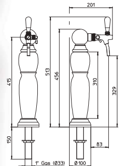
VANITY LEGNO/WOOD C506
