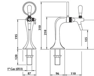
COBRA® PLUS SMALL C104-1 C630-13
