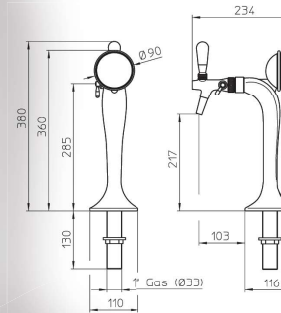
COBRA® PLUS MEDIUM C630-12
